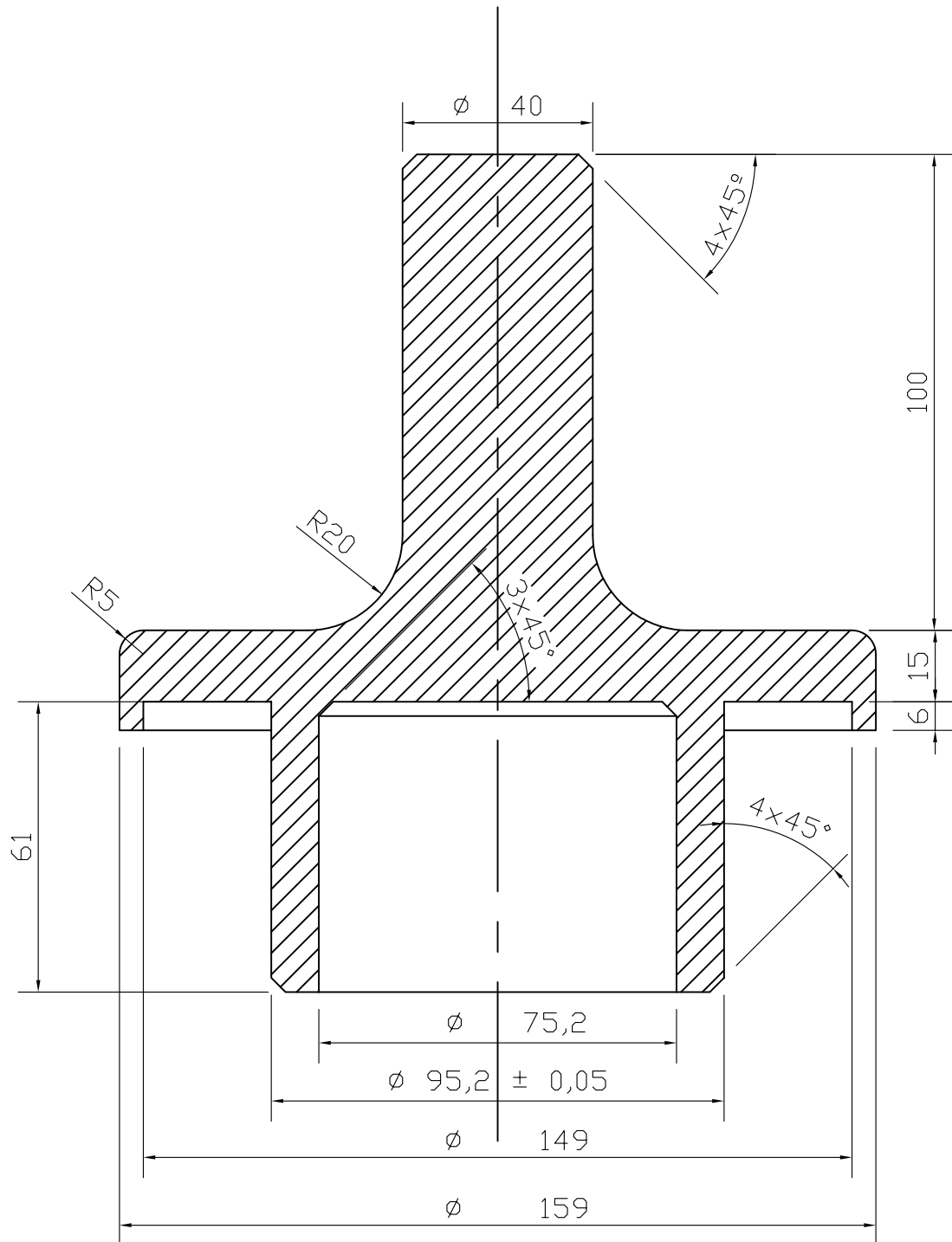
CUBO DE RODA TRASEIRO
